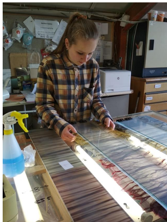
Laminování skla
